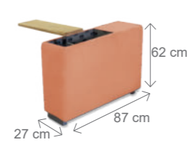
područka USB
